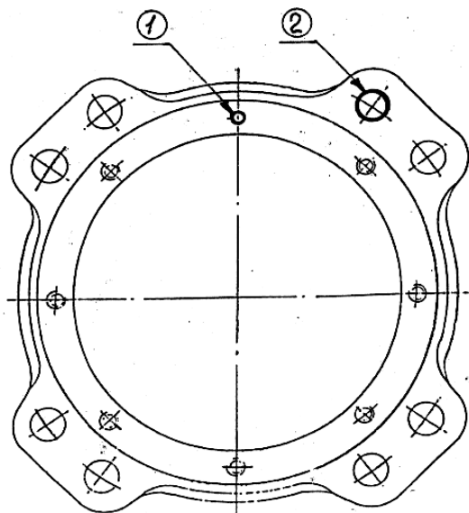
Рисунок 5.12 – Крышка крепительная
