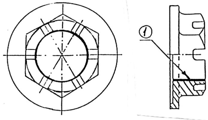
Рисунок 7.14 – Гайка шпинтона
