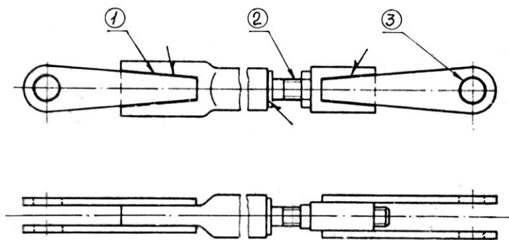
Рисунок 5.169 - Тяга
