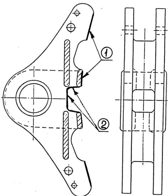
Рисунок 5.34 – Башмак
