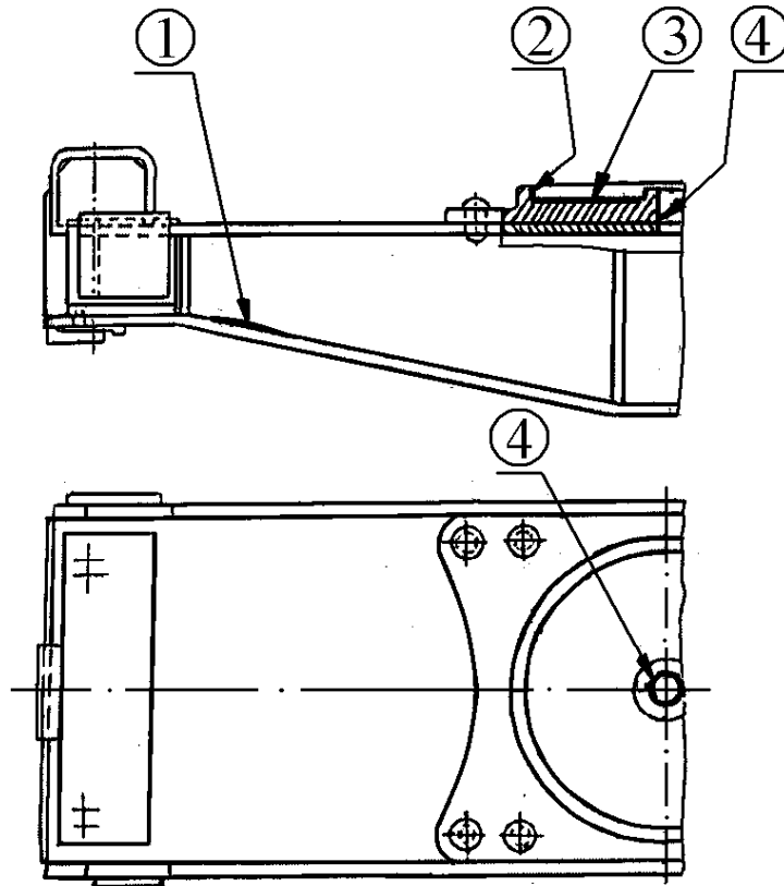
Рисунок 5.17 - Брус надрессорный
