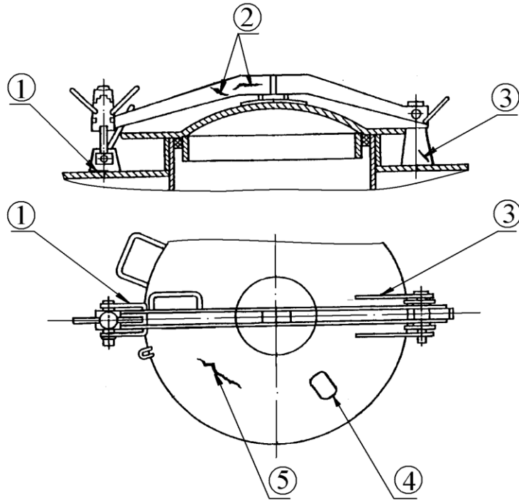
Рисунок 5.136 - Крышка ригельного типа
