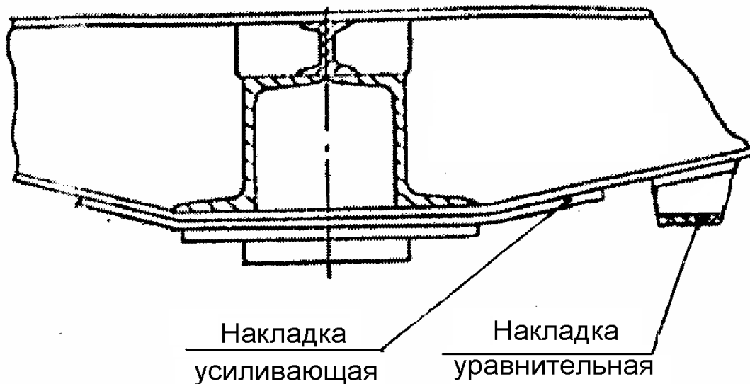
Рисунок 5.71 - Усиление накладкой нижнего листа шкворневой балки полувагона
