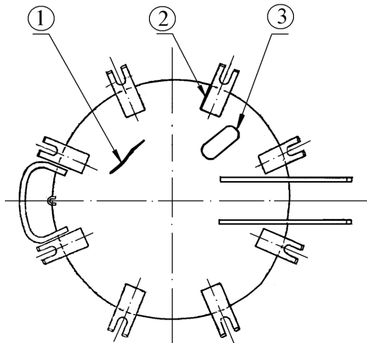
Рисунок 5.135 - Крышка колпака
