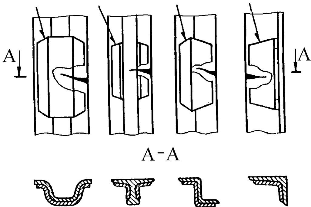
Рисунок 5.75 – Стойки кузова вагона, усиленные профильными накладками
