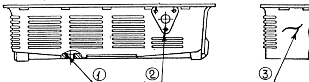
Рисунок 5.95- Ванна масляная
