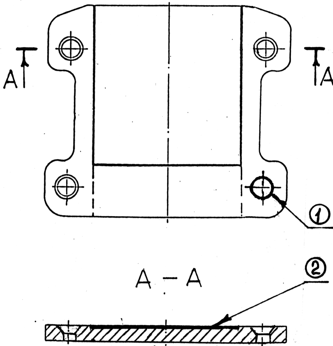
Рисунок 5.8 - Планка фрикционная
