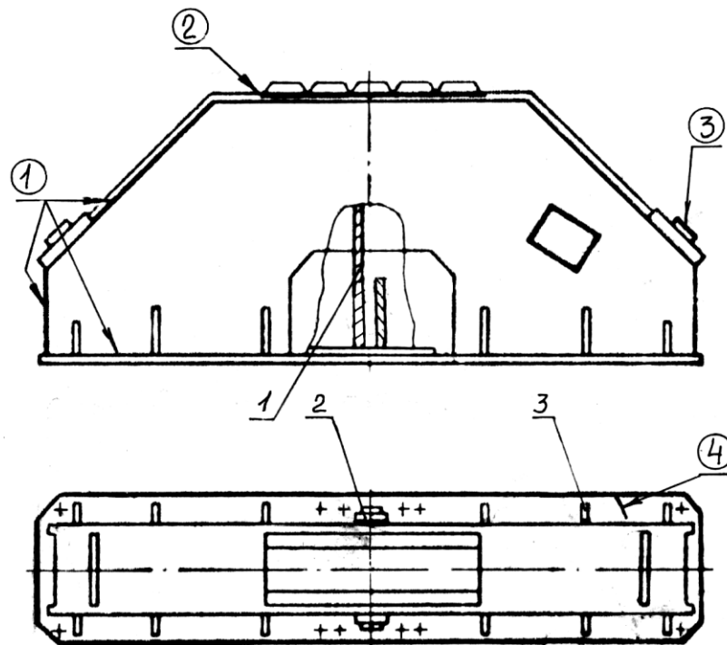
Рисунок 5.148 - Опора
