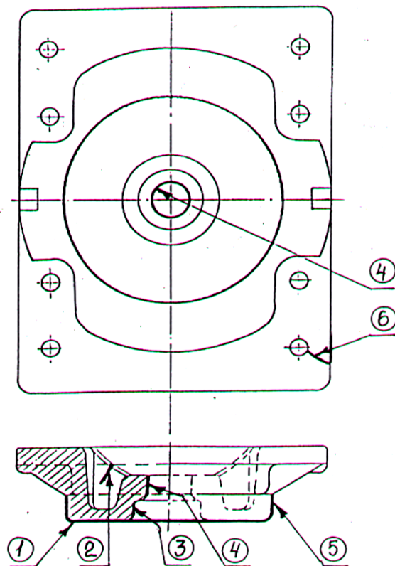
Рисунок 5.73 – Пятник
