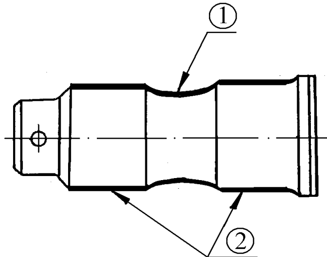
Рисунок 5.16 – Валик
