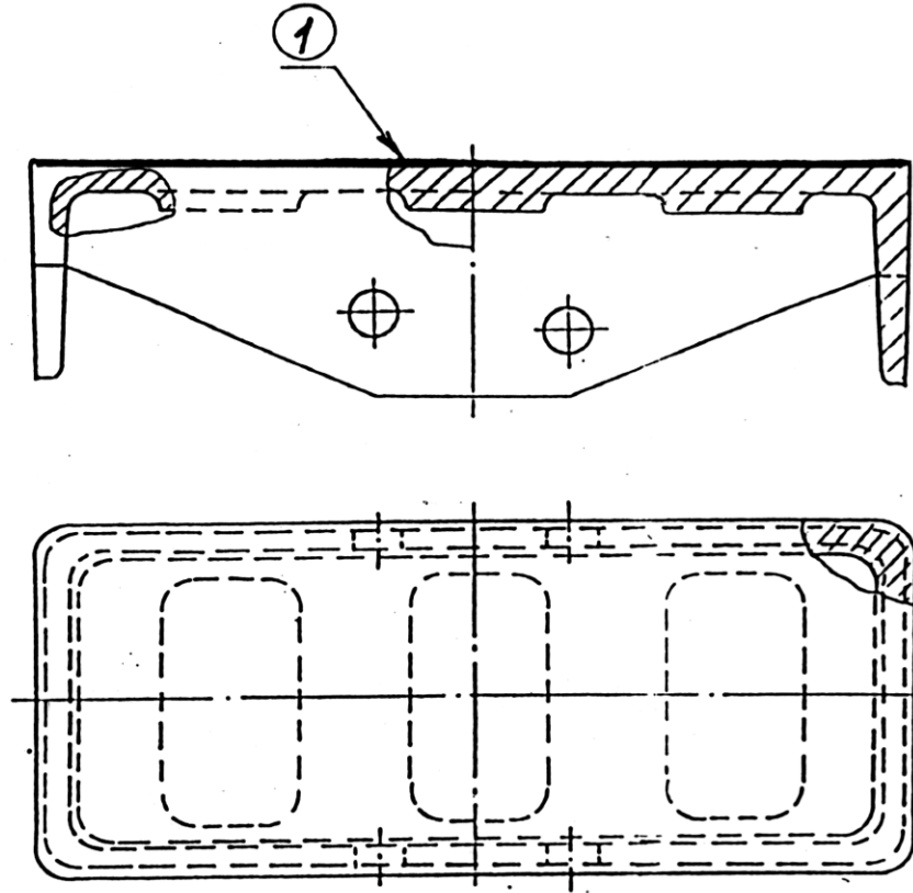
Рисунок 5.10 - Колпак скользуна
