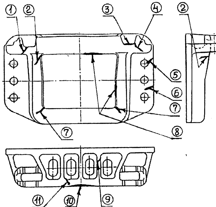
Рисунок 5.47 – Розетка ударная
