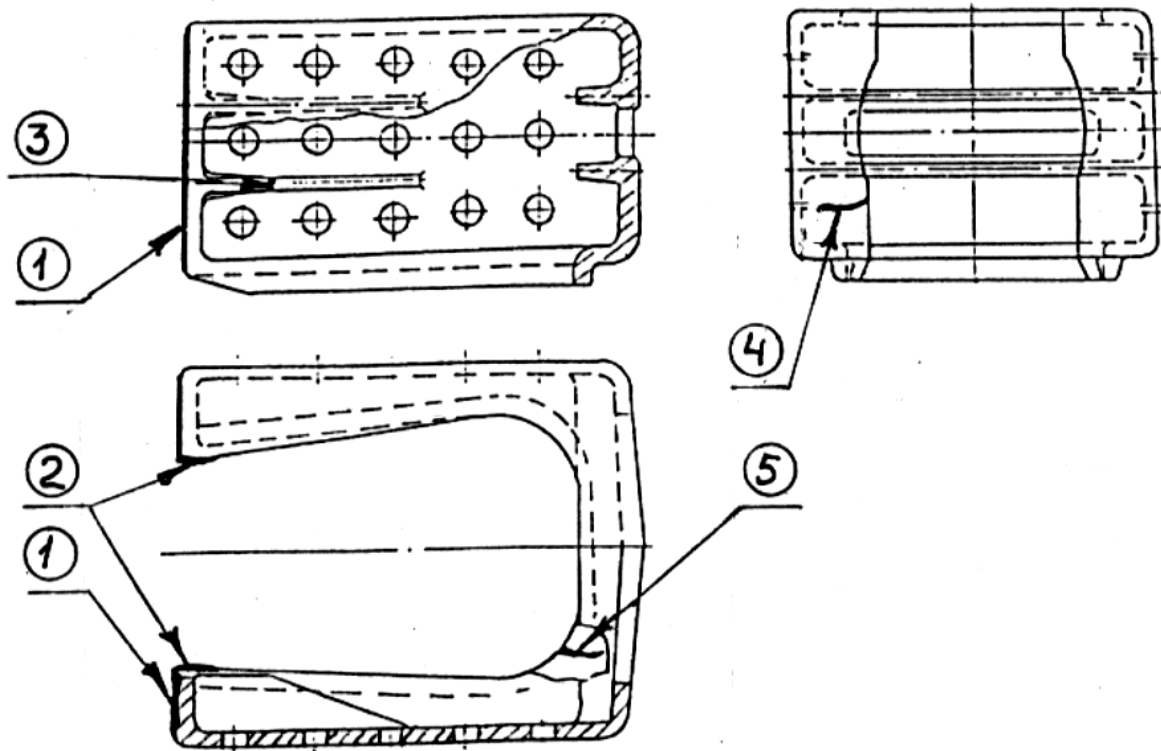
Рисунок 5.59 - Упор задний
