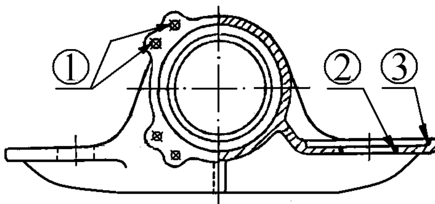
Рисунок 5.11 - Корпус буксы
