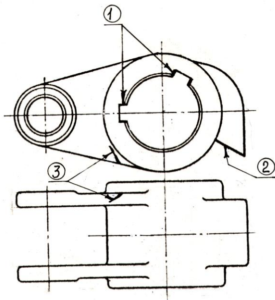
Рисунок 5.175 - Рычаг поворотный
