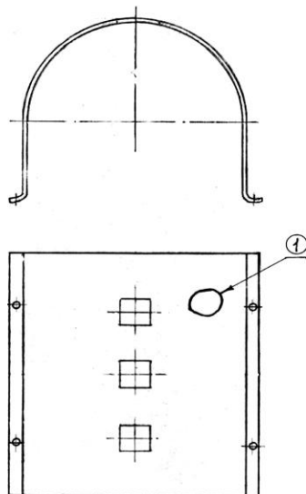
Рисунок 5.180 – Кожух цилиндра
