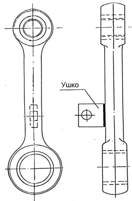
Рисунок 5.35 - Подвеска башмака
