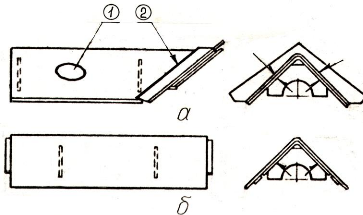
Рисунок 5.167 – Коньки хребтовой балки: а - крайний; б - средний
