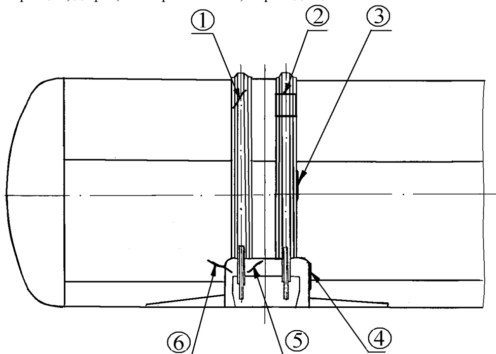
Рисунок 7.133 - Котел восьмиосной цистерны
