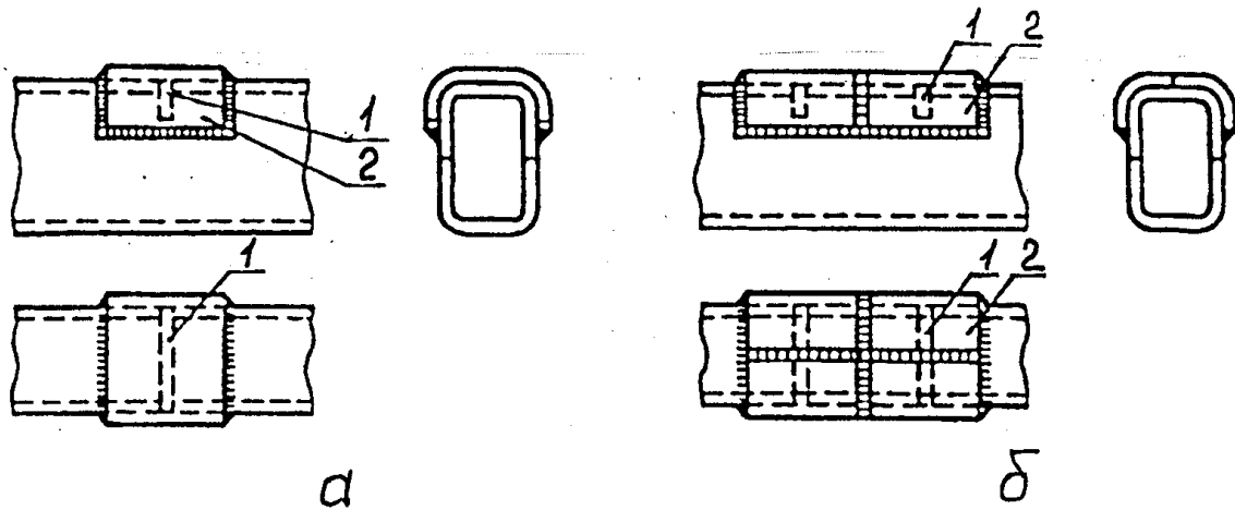
Рисунок 3.3 - Схемы конструктивных усиления после заварки трещин:
