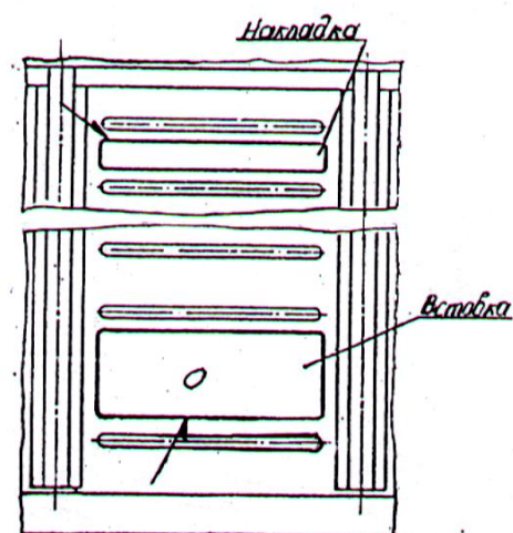
Рисунок 5.81 – Приварка накладки и вставки в межстоечный проем
