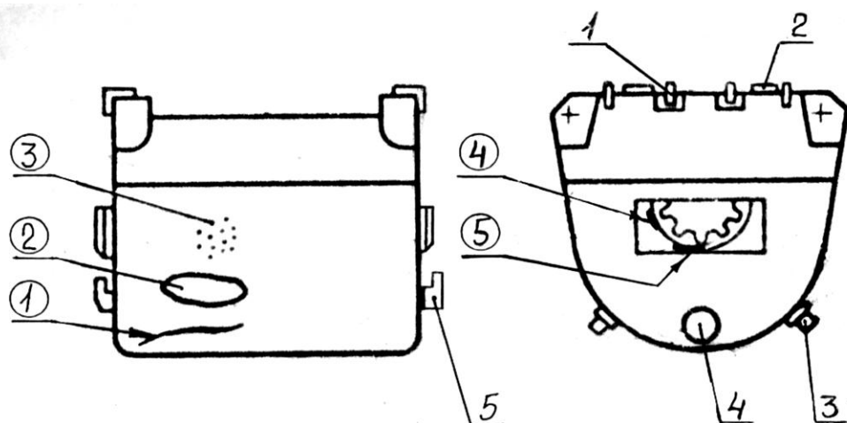
Рисунок 5.147 – Бункер
