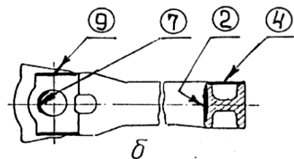
Рисунок 5.57 - Хомут тяговый:
