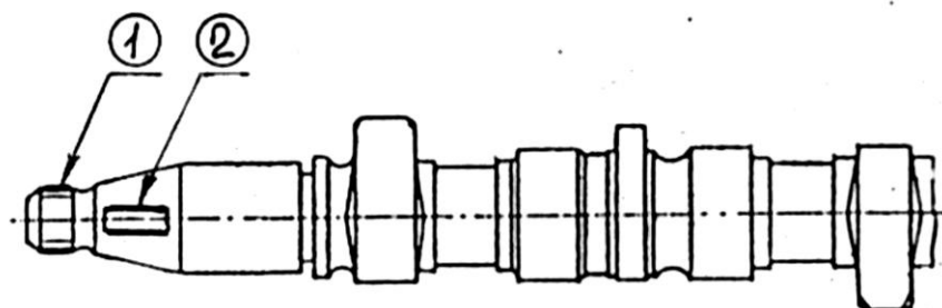
Рисунок 5.101 - Вал кулачковый топливного насоса
