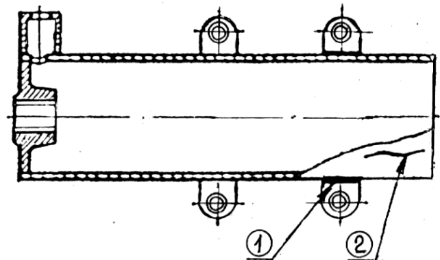
Рисунок 5.120 - Корпус масляного фильтра
