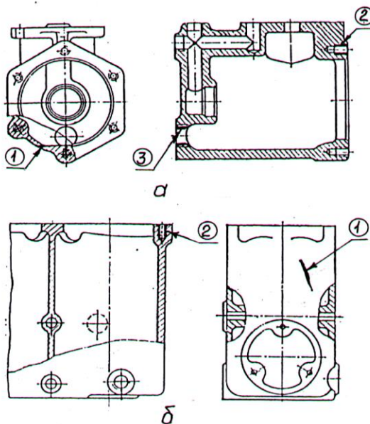
Рисунок 5.94 - Корпус масляного фильтра: а) дизель 4 НБД-12,5; б) дизель 4 ВД-21/15
