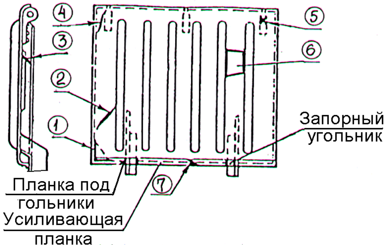
Рисунок 5.83 – Крышка люка полувагона
