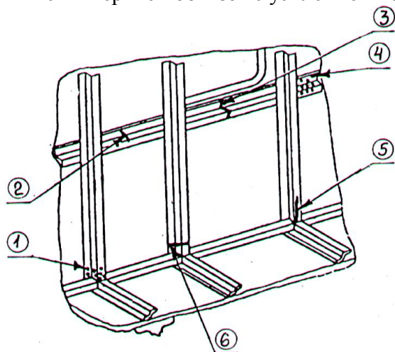
Рисунок 5.76 – Каркас кузова рефрижераторного вагона
