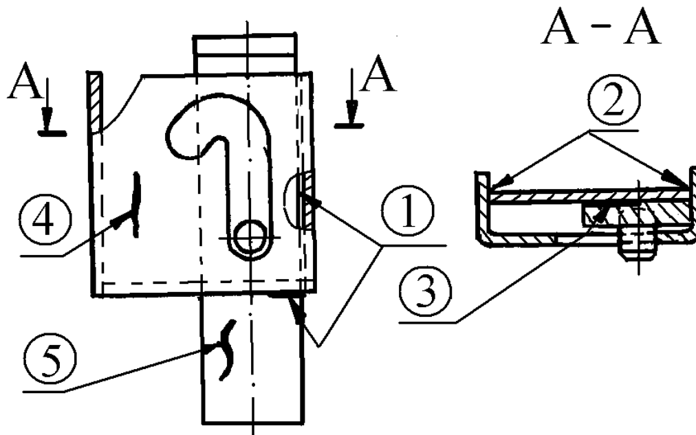
Рисунок 5.87 - Нижний запорный механизм торцевой двери полувагона
