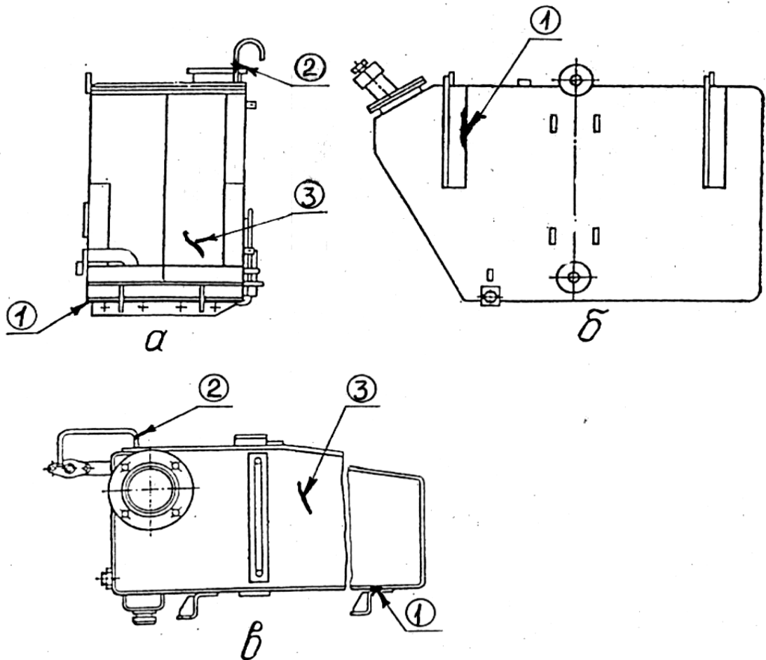
Рисунок 5.129- Бак топливный:
