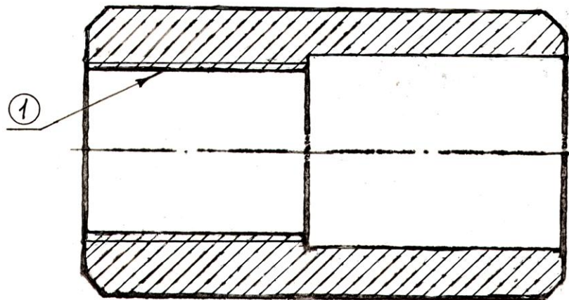
Рисунок 5.161 – Муфта
