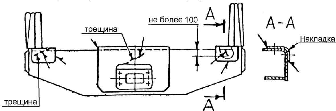
Рисунок 5.67 - Балка полувагона с металлической обшивкой, отремонтированная сваркой
