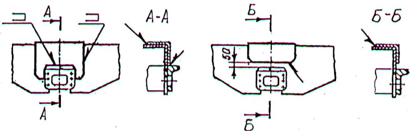
Рисунок 5.64 - Постановка накладки на балке над ударной розеткой
