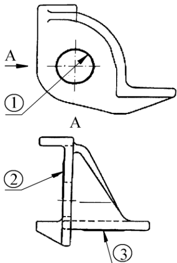
Рисунок 5.30 - Наконечник триангеля
