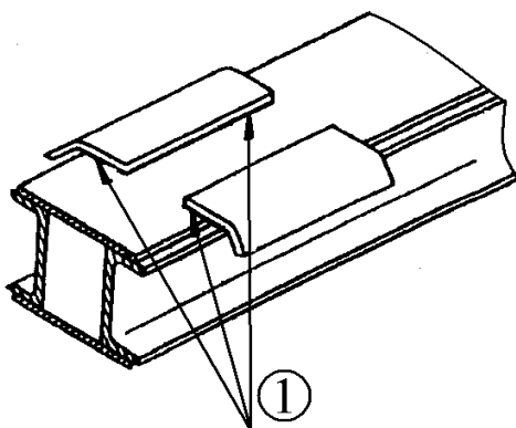
Рисунок 5.139 - Опорная планка
