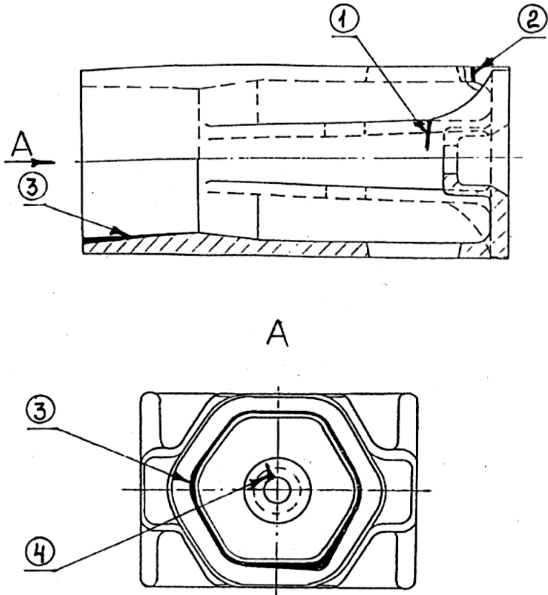
Рисунок 5.52 - Корпус поглощающего аппарата
