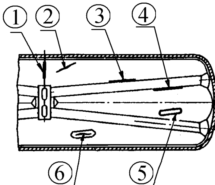
Рисунок 5.145 - Устройство аэропневмовыгрузки
