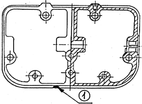
Рисунок 5.113 – Кронштейн коромысла
