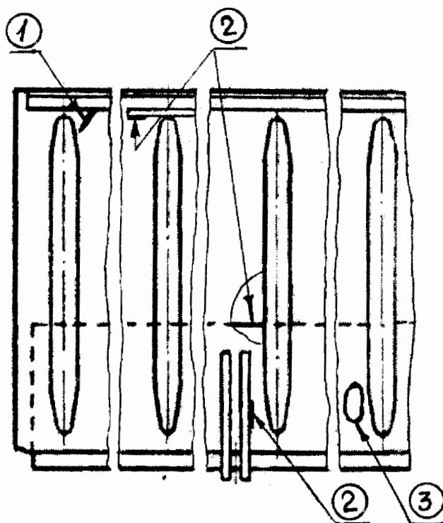
Рисунок 5.153 – Крышка разгрузочного люка
