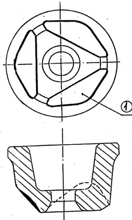
Рисунок 5.53 - Конус нажимной
