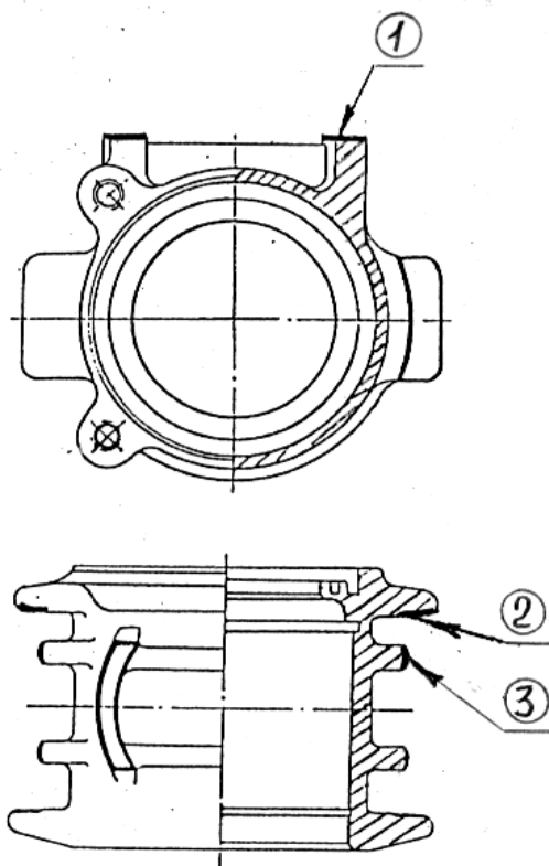
Рисунок 5.4 - Корпус буксы
