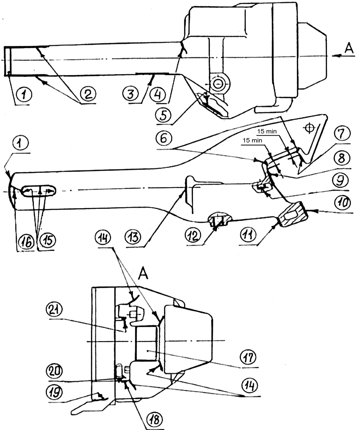
Рисунок 5.41 Корпус автосцепки
