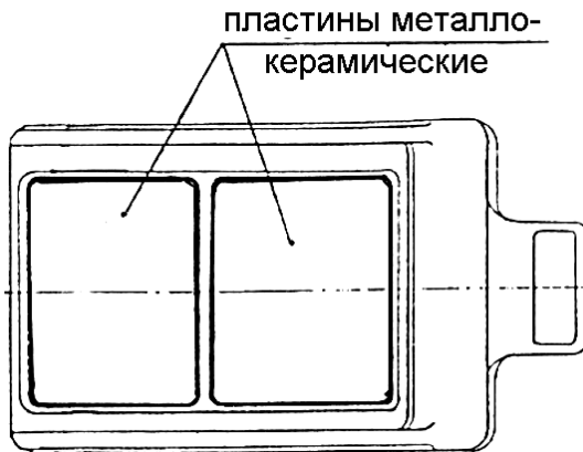
Рисунок 5.55 - Пластина неподвижная
