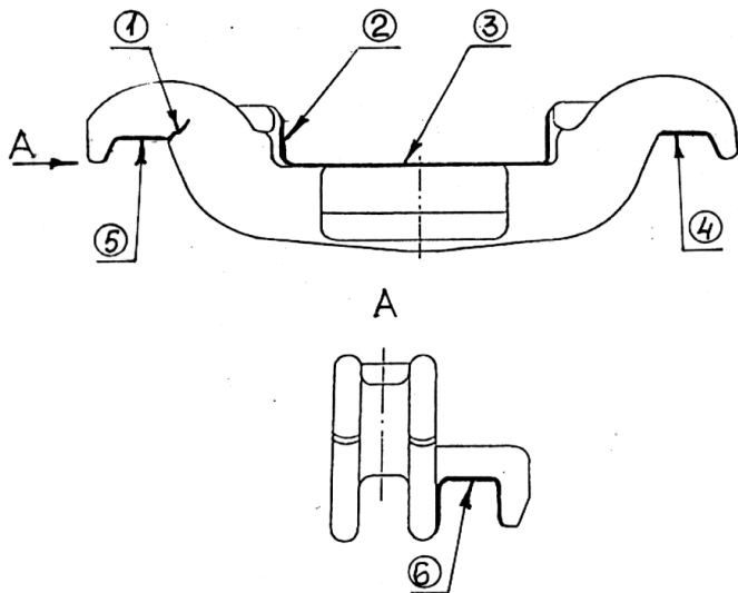
Рисунок 5.48 - Балочка центрирующая
