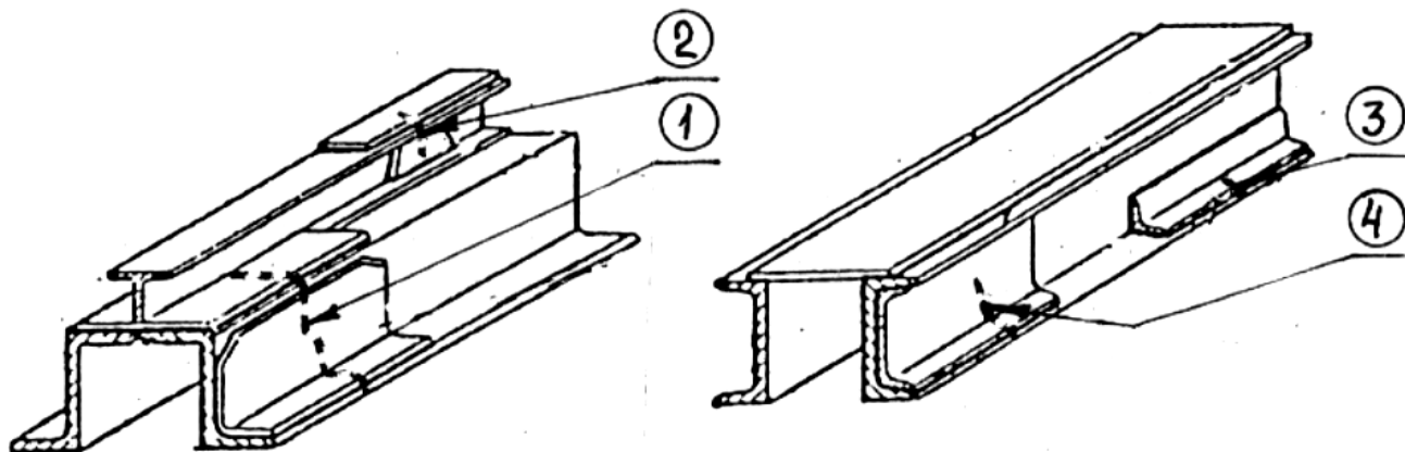
Рисунок 5.62 - Балки хребтовые с трещинами и изломами, отремонтированные накладками
