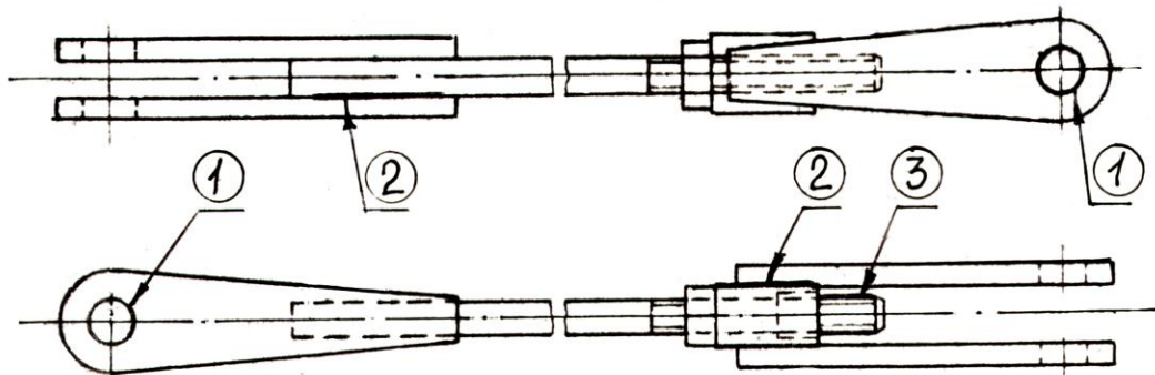
Рисунок 5.184 - Тяга
