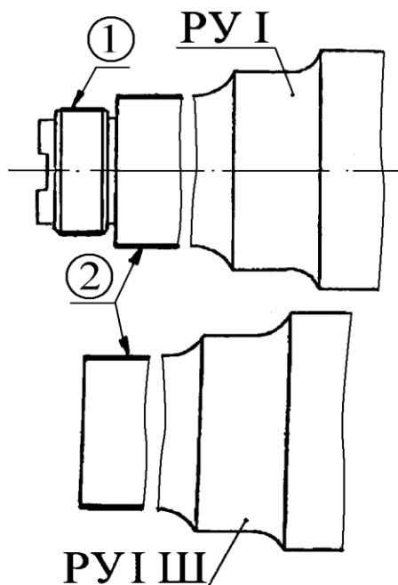
Рисунок 5.1 - Ось
