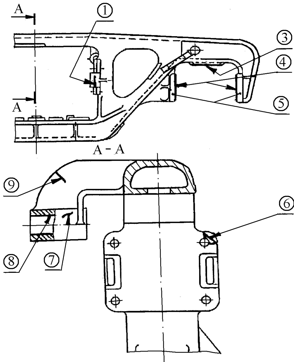
Рисунок 5.7 - Рама боковая
