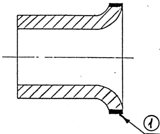
Рисунок 5.40 Втулка упорная регулятора 74 Б
