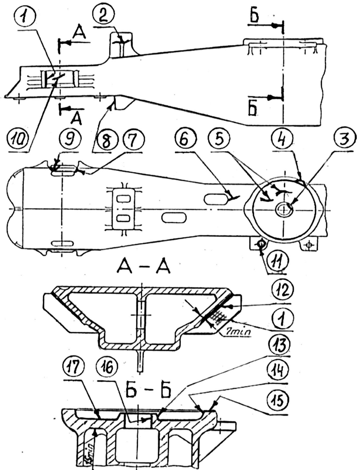
Рисунок 5.5 - Балка надрессорная
