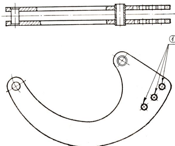
Рисунок 5.164 - Рычаг двулучный
