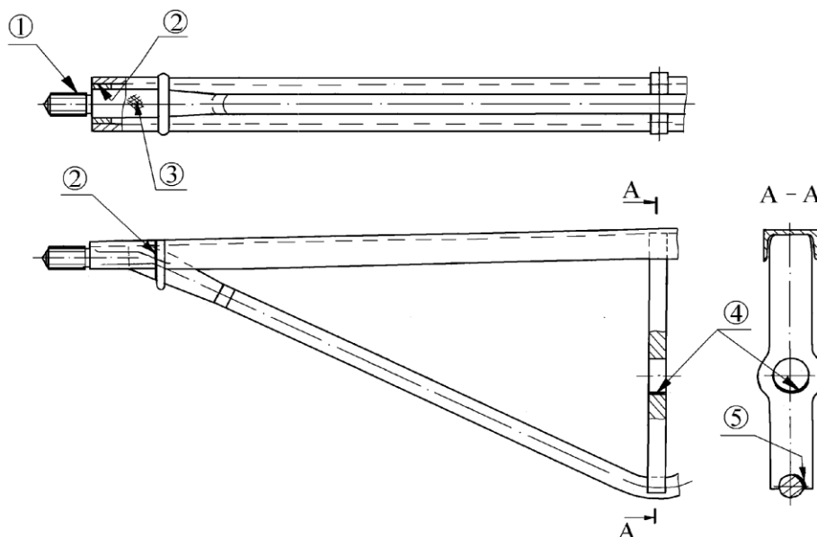
Рисунок 5.29 - Балка триангеля со струной и распоркой
