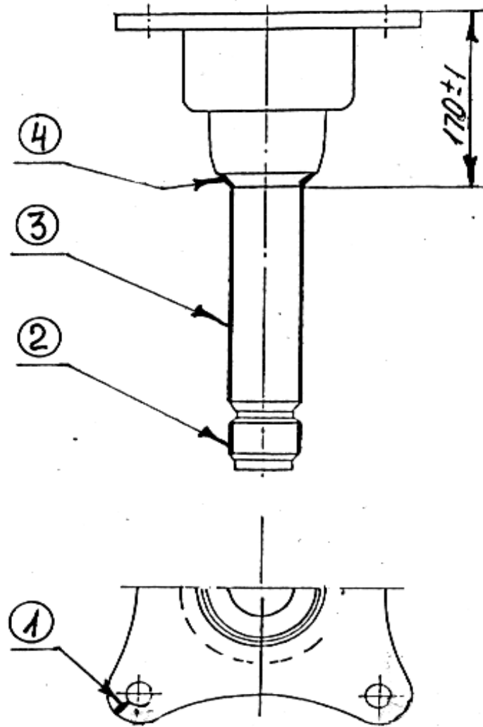
Рисунок 5.13– Шпинтон
