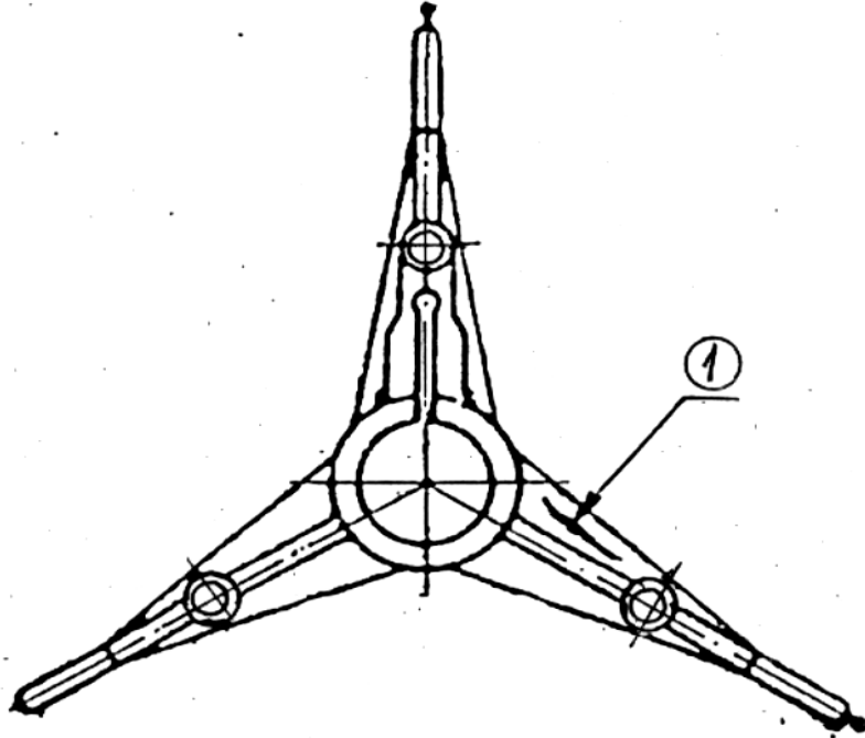
Рисунок 5.124 - Вентилятор асинхронного двигателя
