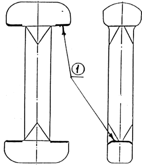
Рисунок 5.49 – Подвеска маятниковая
