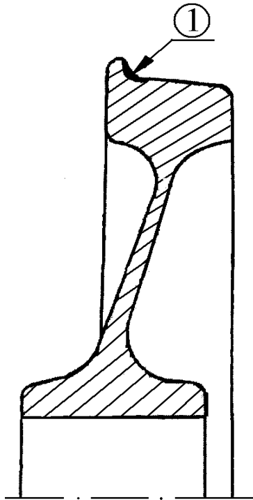
Рисунок 5.2 - Колесо цельнокатаное
