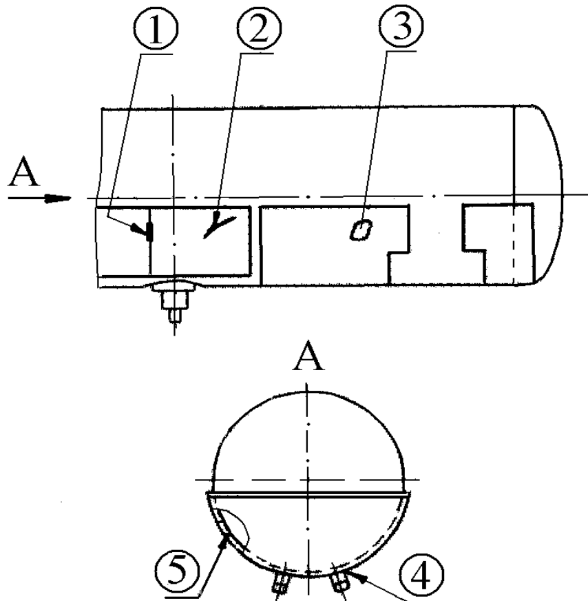
Рисунок 5.142 - Паровая рубашка котла
