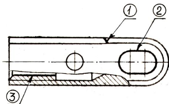
Рисунок 5.182 - Головка штока
