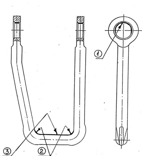
Рисунок 5.32 – Подвеска триангеля
