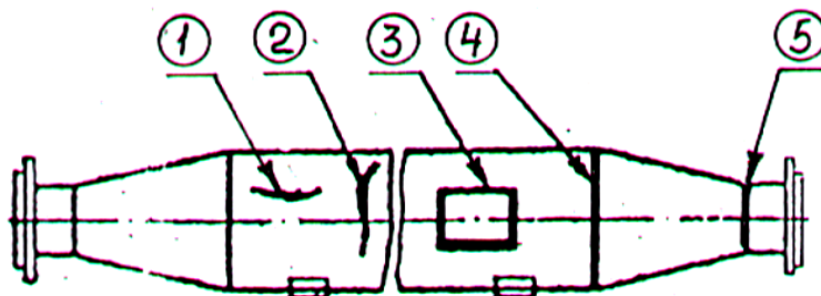
Рисунок 5.93 - Глушитель
