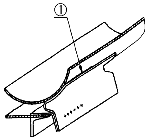
Рисунок 5.138 – Узел крепления котла к хребтовой балке
