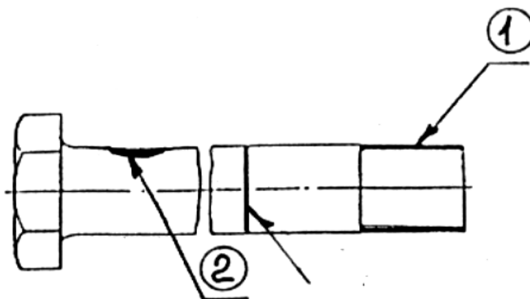
Рисунок 5.51 – Болт стяжной
