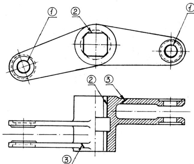
Рисунок 5.178– Вилка поворотная
