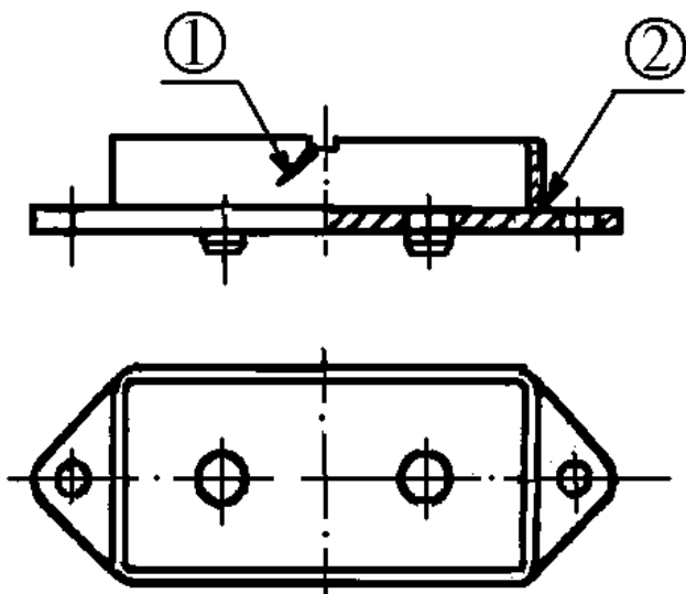
Рисунок 5.19 - Коробка скользя
