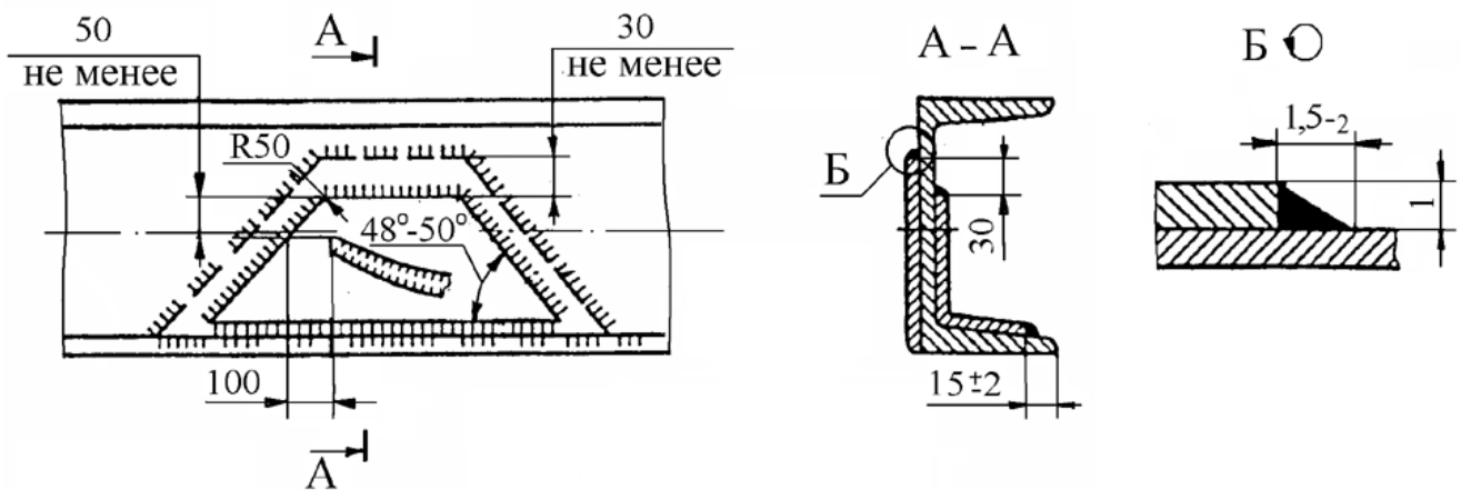
Рисунок 3.4 - Приварка двусторонних накладок со смещением противоположных швов
