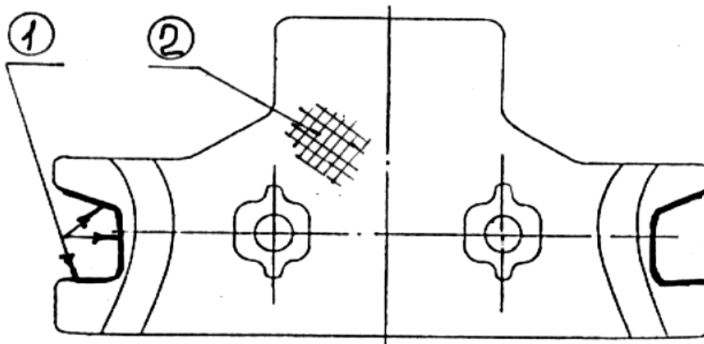
Рисунок 5.50 - Плита поддерживающая
