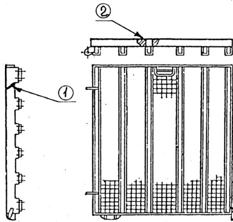
Рисунок 5.128- Решетка напольная
