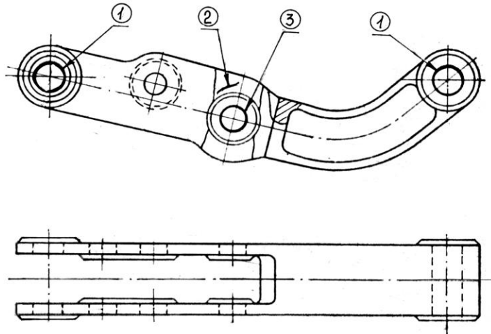
Рисунок 5.179 – Рычаг
