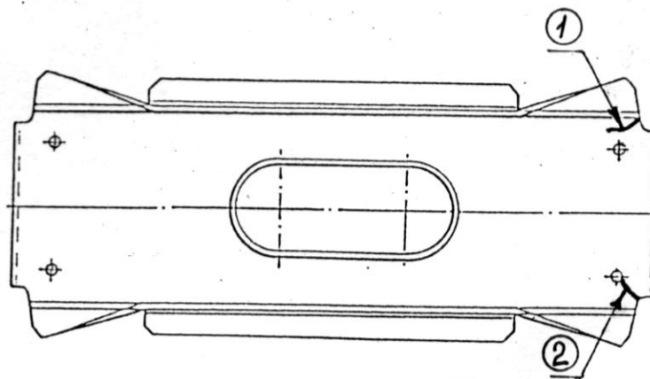
Рисунок 5.18 - Брус подрессорный
