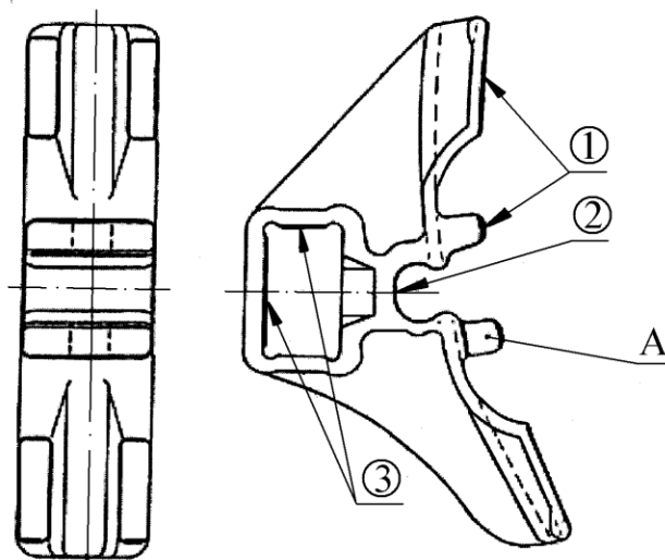
Рисунок 5.31 - Башмак неповоротный
