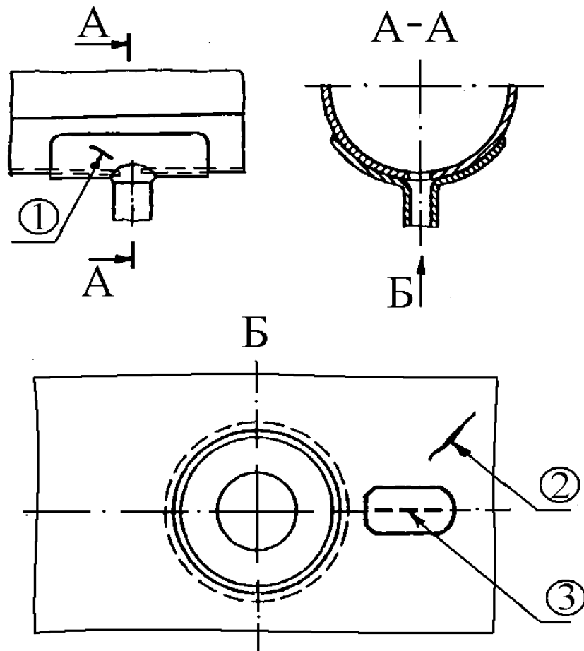
Рисунок 5.132 - Броневой лист
