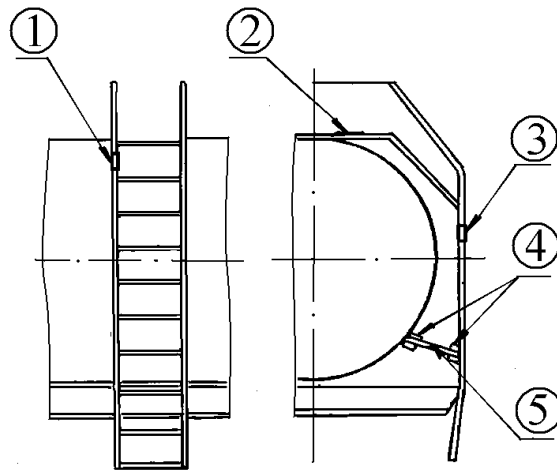
Рисунок 5.141 - Наружная лестница
