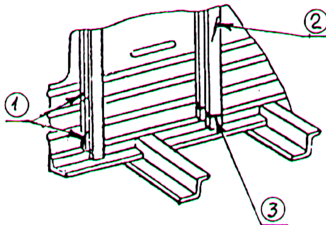
Рисунок 5.77- Боковые стойки рефрижераторного вагона
