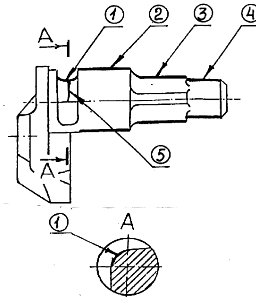
Рисунок 5.46 – Валик подъемника
