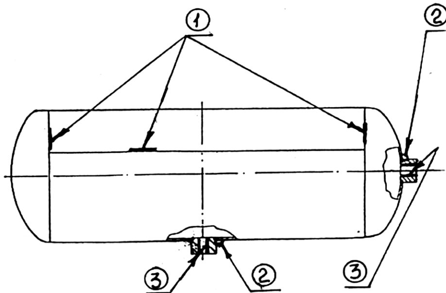
Рисунок 5.25 – Резервуар воздушный
