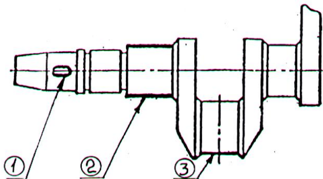
Рисунок 5.91 – Вал коленчатый
