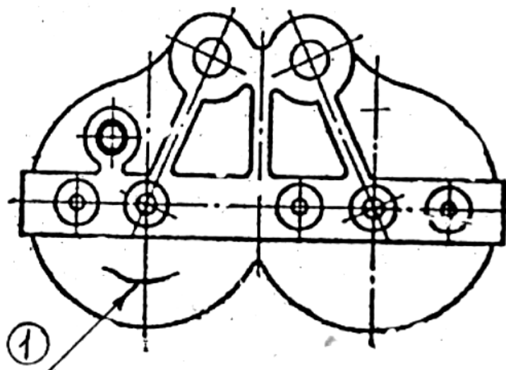
Рисунок 5.102 - Крышка топливного фильтра
