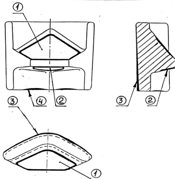
Рисунок 5.54 - Клин фрикционный
