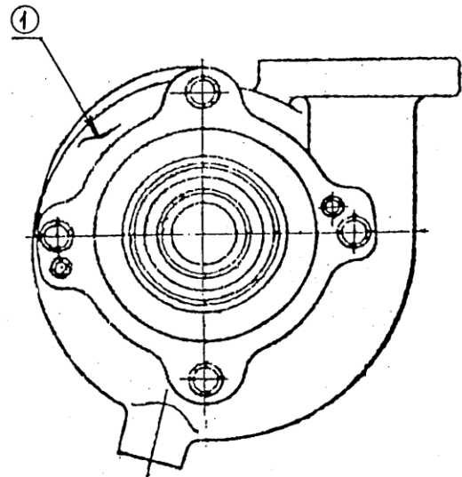
Рисунок 5.118 – Корпус центробежного водяного насоса
