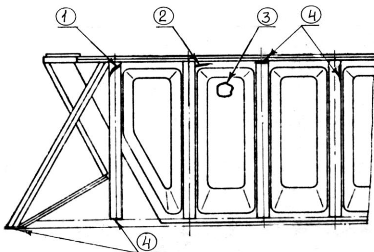
Рисунок 5.149 - Кузов
