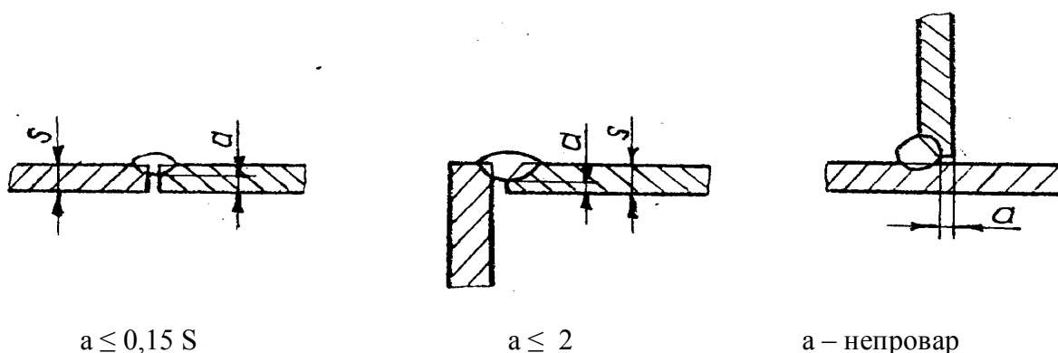
Рисунок 3.1 - Допустимая величина непровара
