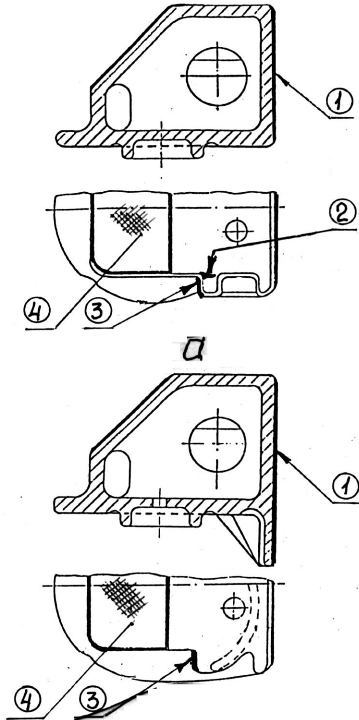
Рисунок 5.9 – Клин а - чертеж 100.30.001-0; б - чертеж 100.30.001-1
