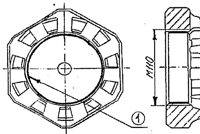
Рисунок 5.3 – Гайка
