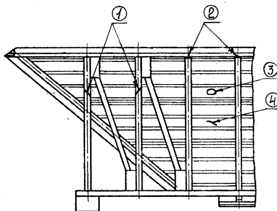
Рисунок 5.166 - Кузов
