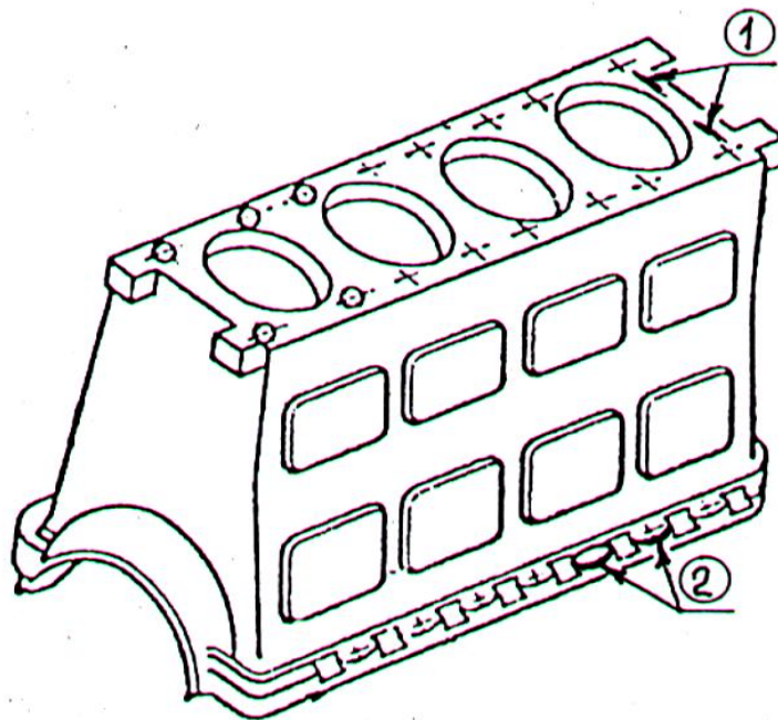
Рисунок 5.88 – Блок цилиндров
