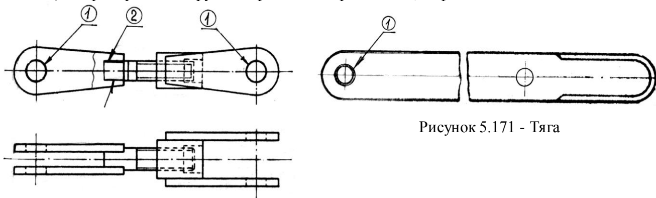
Рисунок 5.170 – Рычаг
