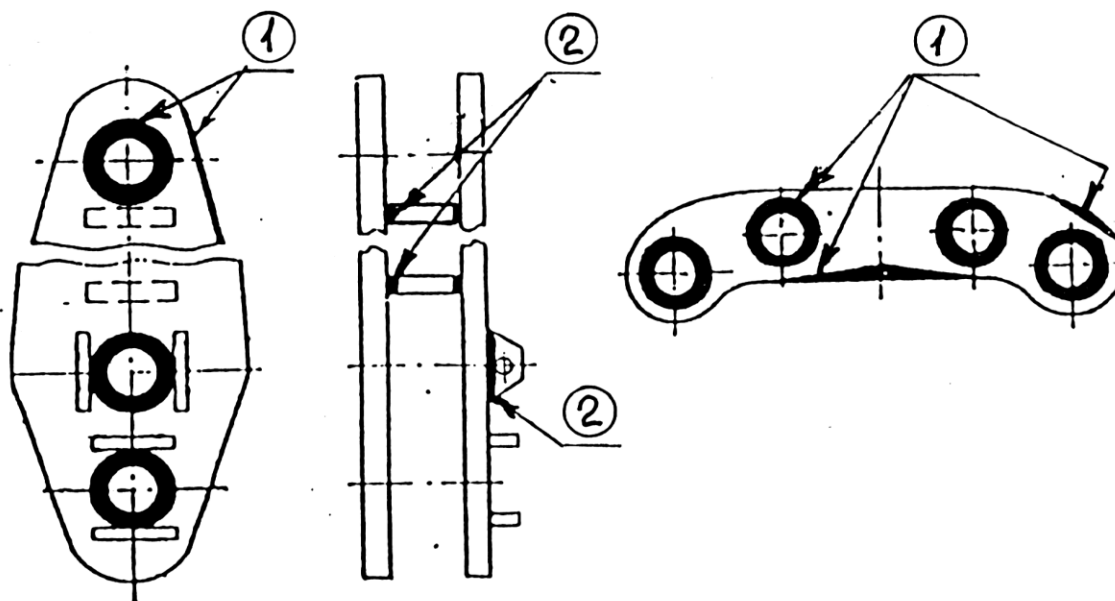
Рисунок 5.36 - Рычаги тормозные и затяжки рычагов
