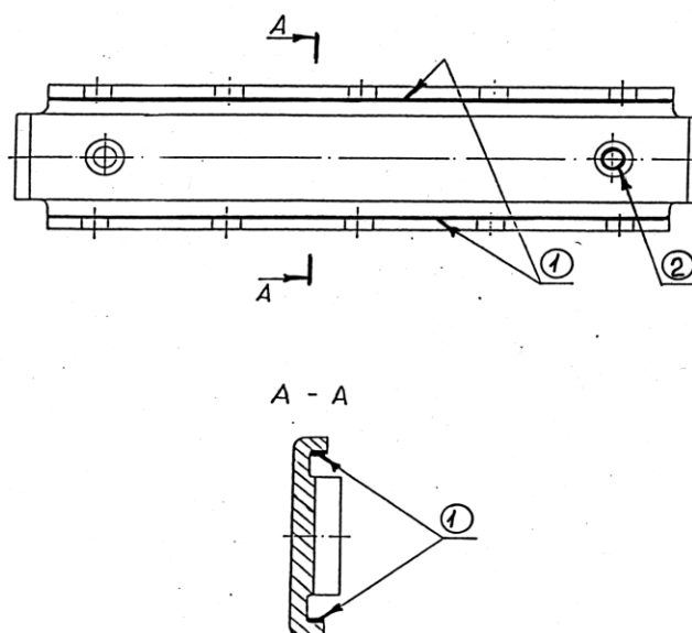
Рисунок 5.23 – Планка рессорная
