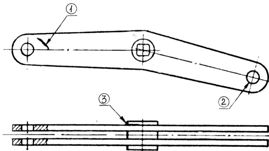
Рисунок 5.162 – Рычаг
