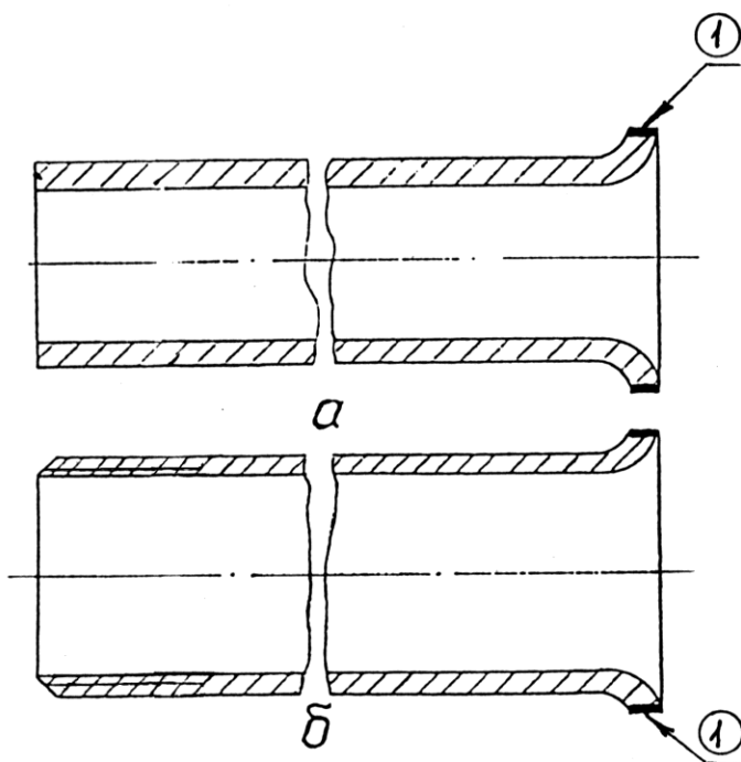
Рисунок 5.37 – Трубка защитная а - регулятора №536Г; б – регуляторов №574Б; РТРП-675
