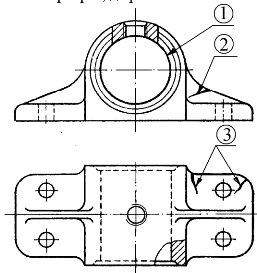
Рисунок 5.174 – Подшипник
