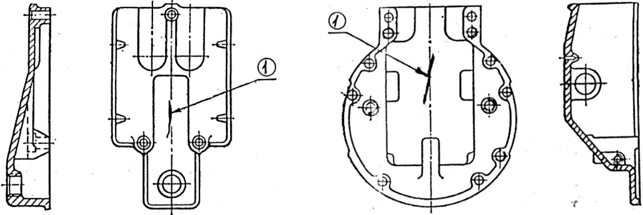
Рисунок 5.108 – Крышка верхняя регулятора оборотов
