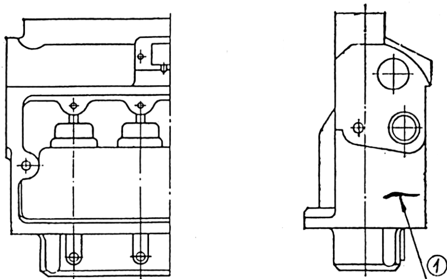
Рисунок 5.99 – Корпус топливного насоса
