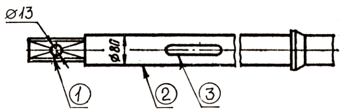
Рисунок 5.158 - Вал
