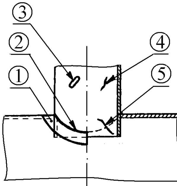
Рисунок 5.134 - Колпак цистерн
