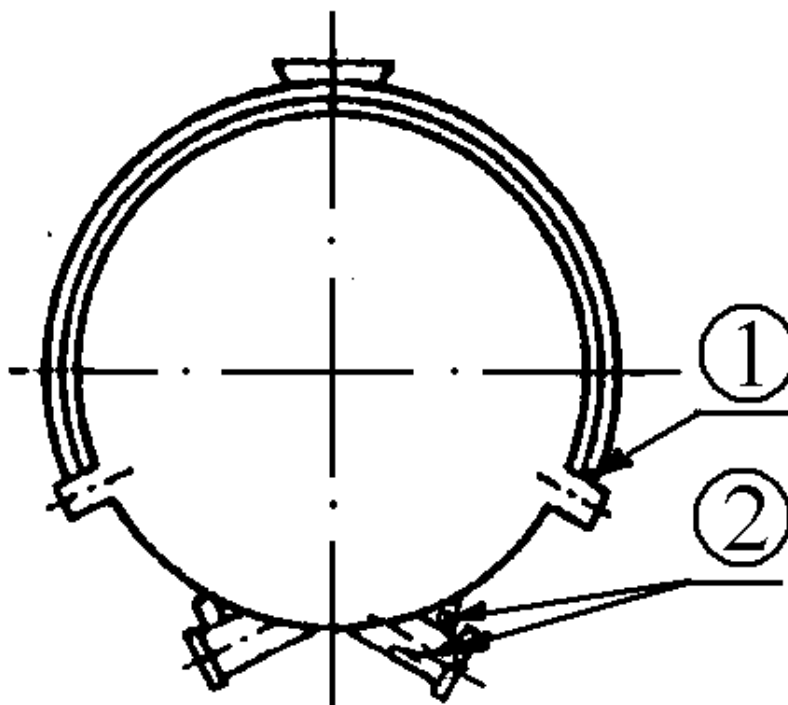
Рисунок 5.144-Разгрузочное устройство
