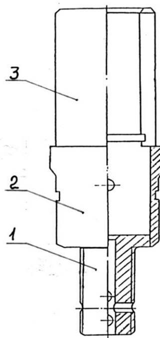
Рисунок 5.38 - Вилка регулятора 1 - труба; 2 - наконечник; 3 - вилка. №265А и 265АI
