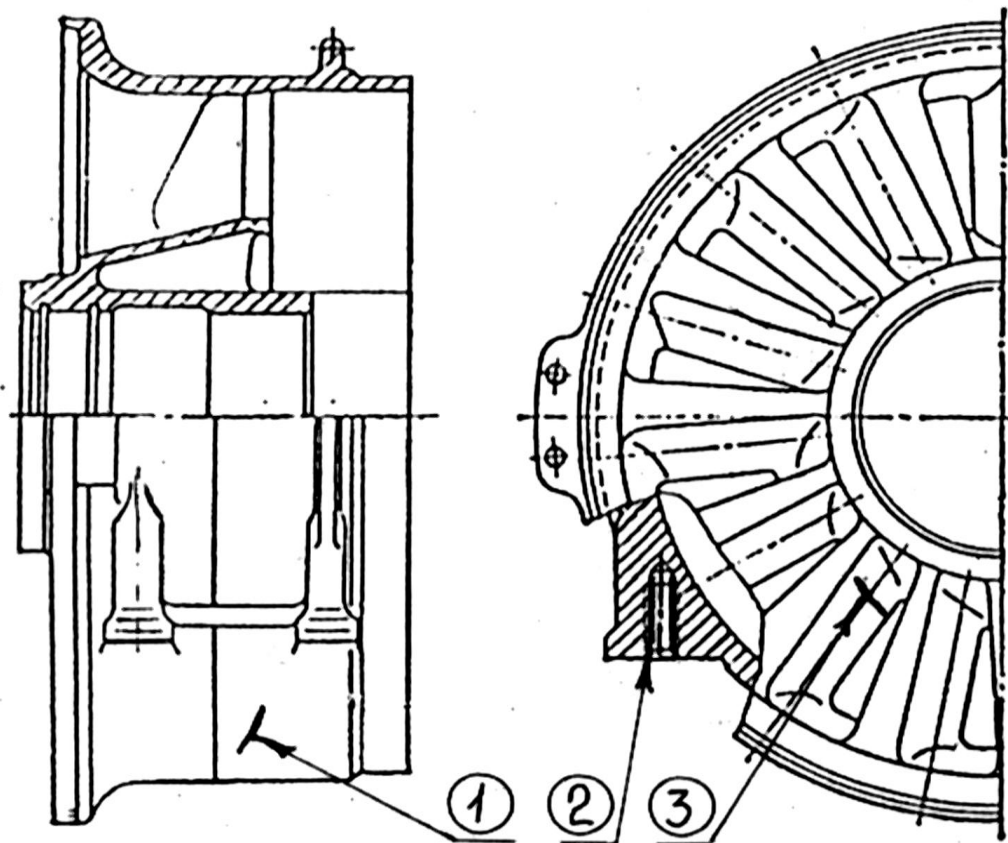
Рисунок 5.96 – Устройство воздуонравляющее
