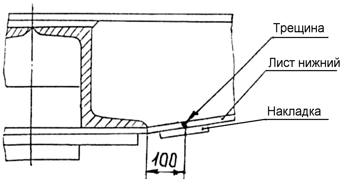
Рисунок 5.70 - Нижний лист шкворневой балки, отремонтированный сваркой
