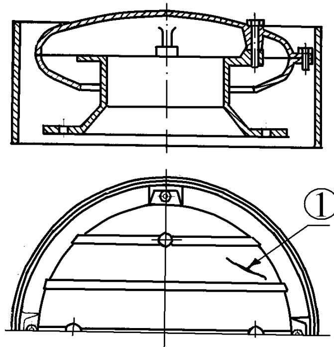
Рисунок 5.126 - Дефлектор
